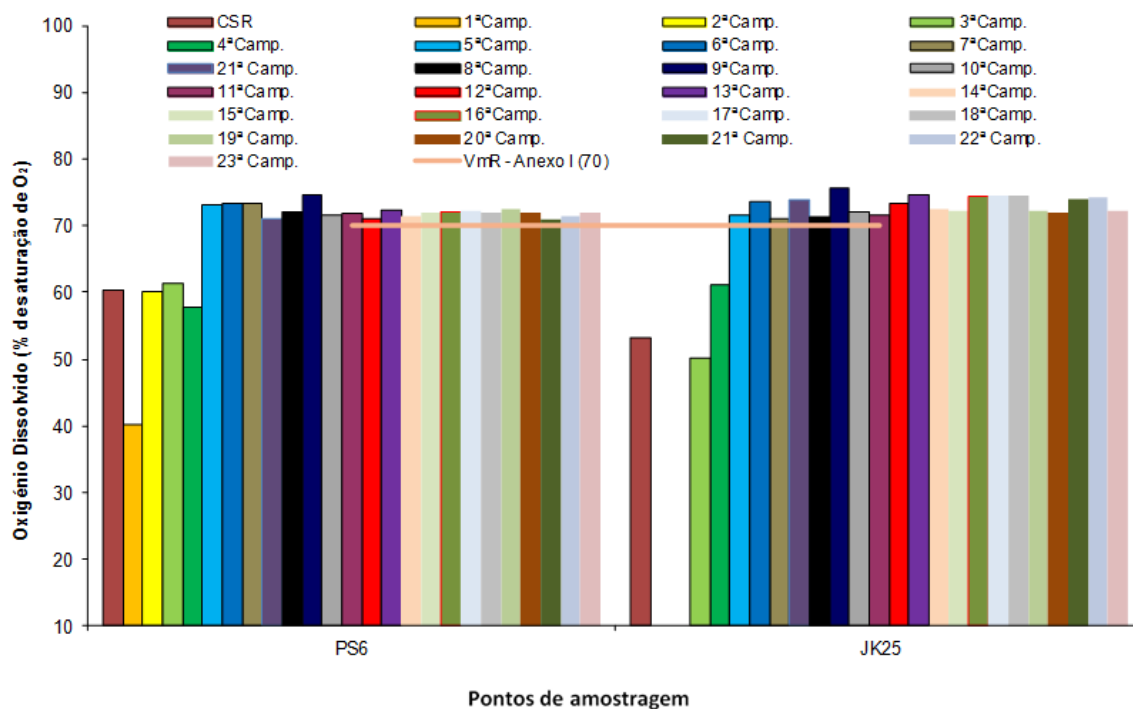
Gráfico 4: Comparação do valor de Oxigénio Dissolvido obtido nas campanhas de monitorização
